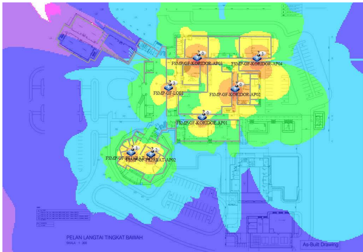
ARAS BAWAH
