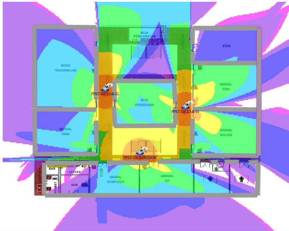
ARAS BAWAH
