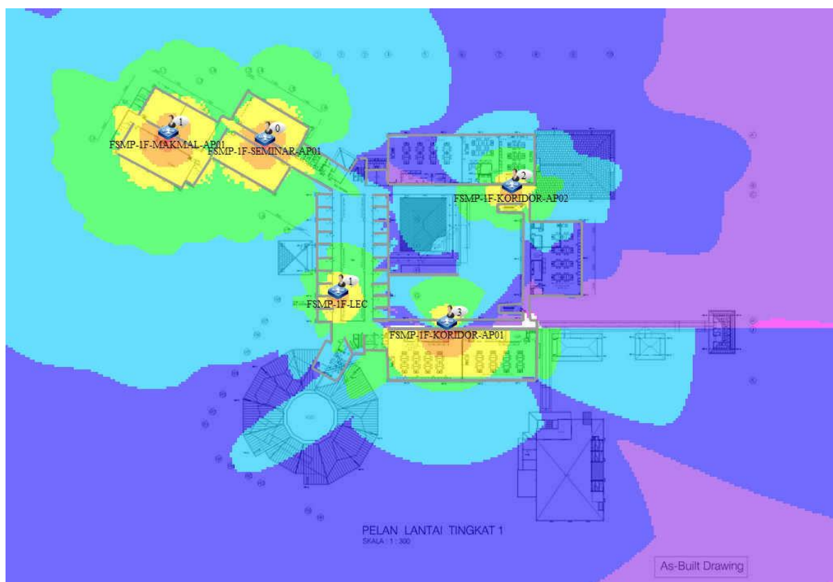
ARAS SATU
