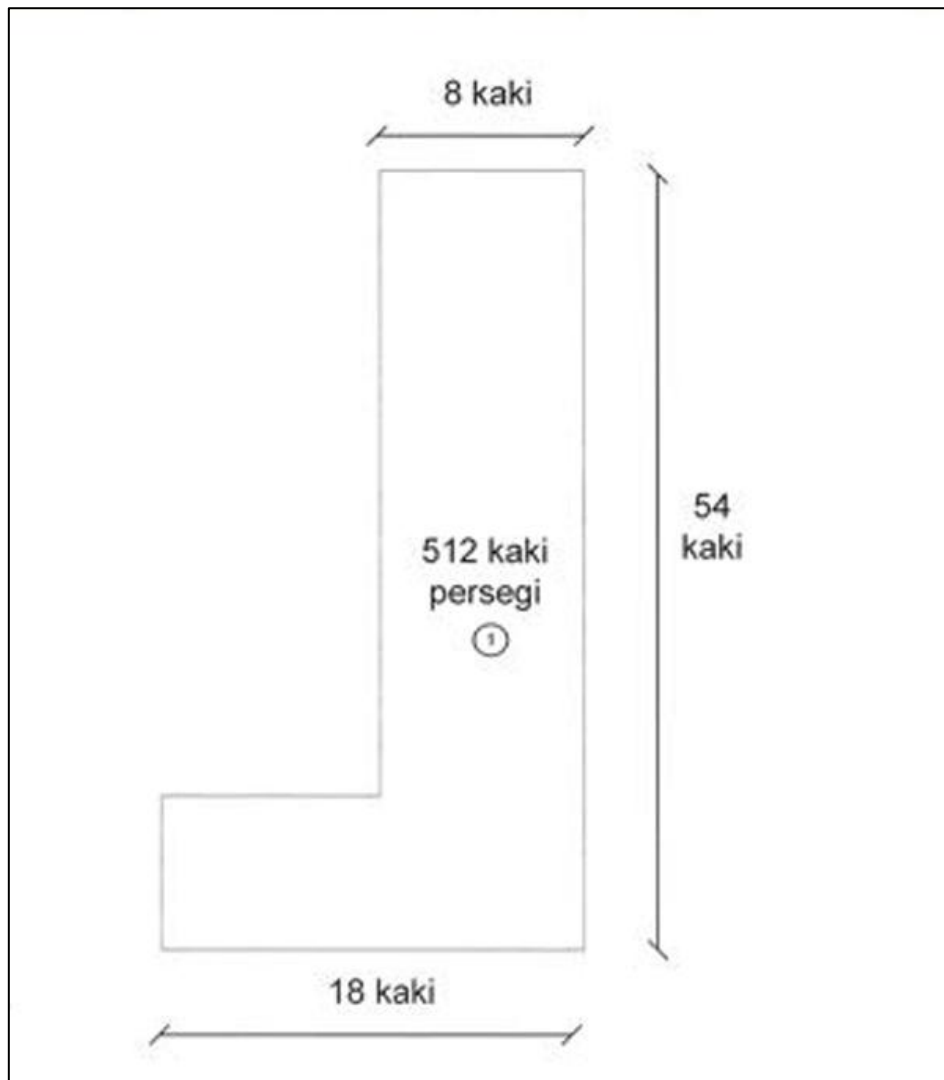
Gambar 4 : Pelan Lantai Kedai Cenderahati
